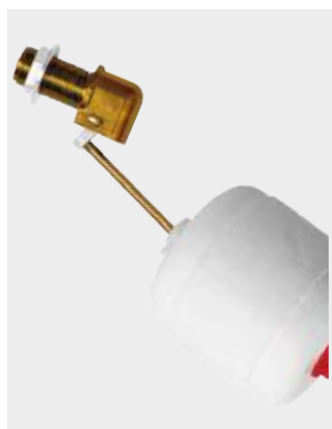
GCB 1 Ref. 0151650630 Packaging Bolsa 25 uds/caja PVP: 8,02 € Grifo lateral (Latón) + Tuerca + Boya Ø 3/8" Latón + Longitud: 30 mm
