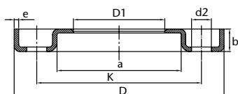
BRIDA PRENSADA
