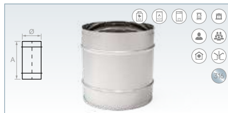
Adaptador Macho - Macho (Acero Inox 316)
